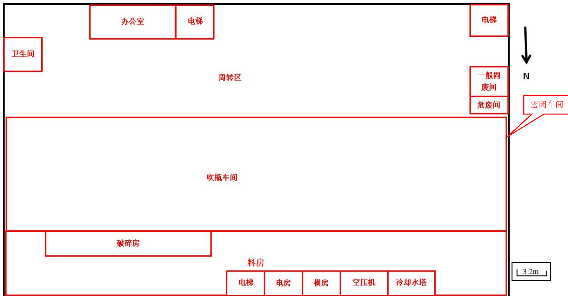
附图 4-1 项目 1F 车间平面布置图
