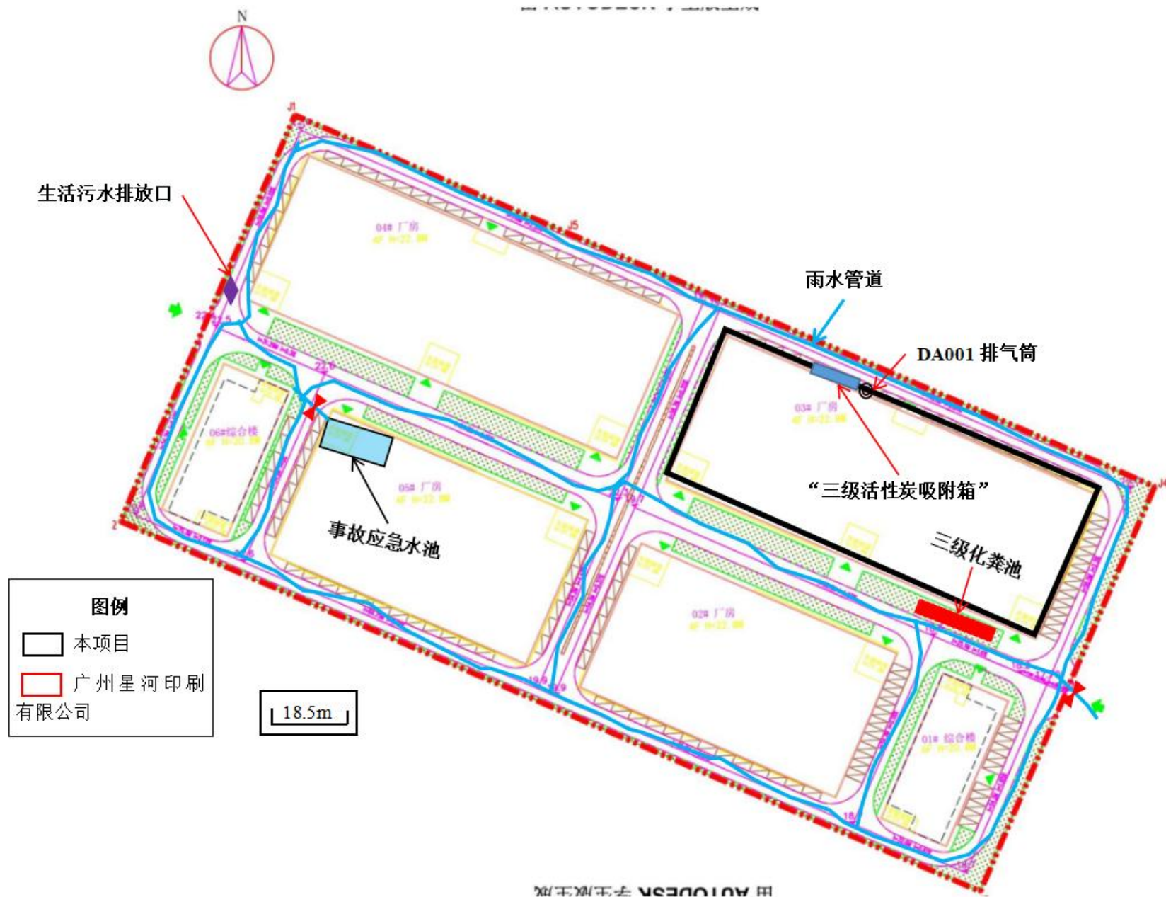
附图 5 项目总平面布置图
