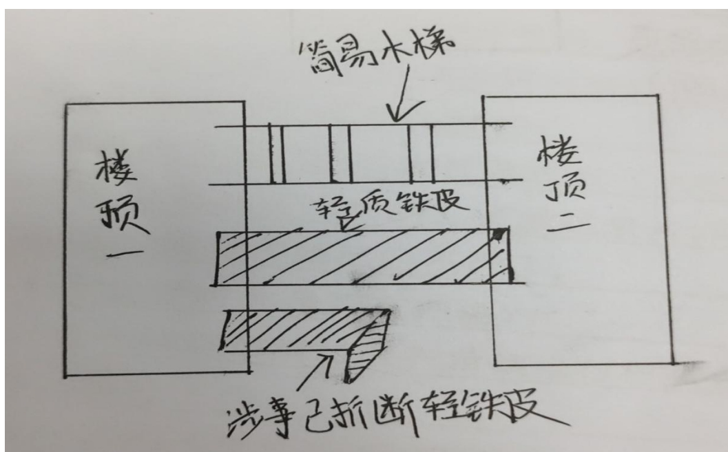
(图三 现场平面图)
