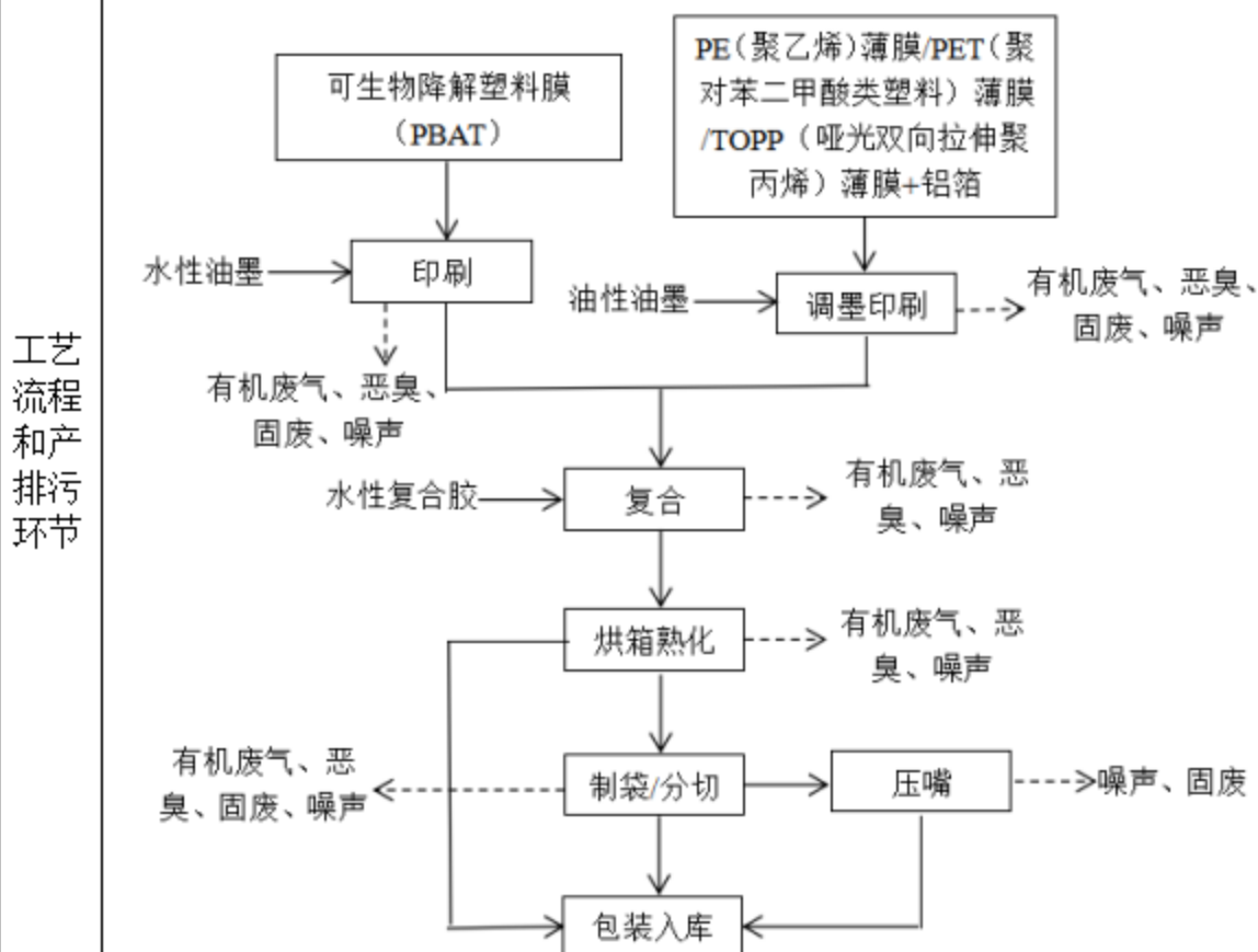
图 3 项目生产工艺流程图
