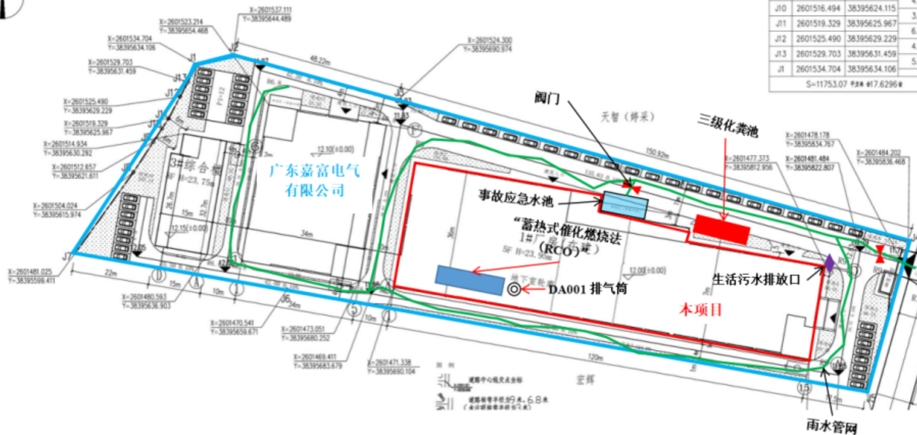
附图 5 项目总平面布置图
