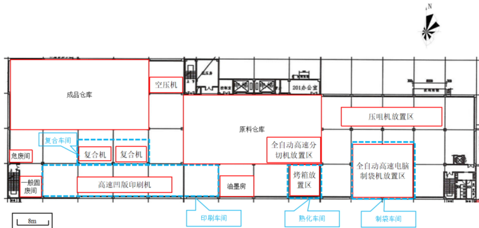
附图 4 项目车间平面布置图
