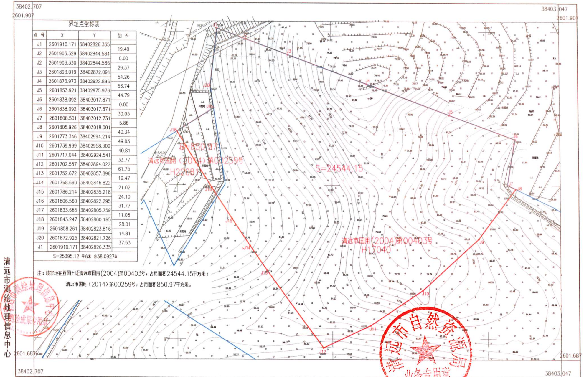
441802007013GB01287用地平面图
